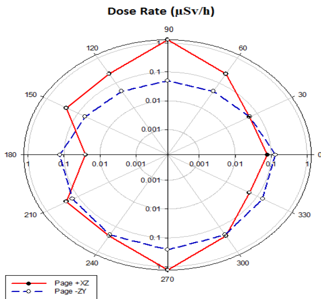
منحنی آهنگ دز برای شاتر بسته سزیم 100 mCi
