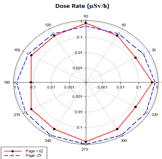
منحنی آهنگ دز برای شاتر بسته کبالت 1 mCi
